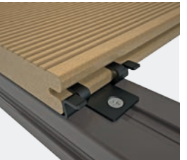
Výr. č. 9477 Montážna svorka pre systém Terrace Massive a Terrace Massive Pro vhodná pre materiál Twinson alebo drevený nosný profil
