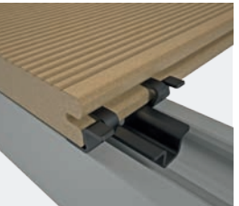
Výr. č. 9365/9467 Montážna svorka pre systém Terrace Massive a Terrace Massive Pro vhodná pre všetky hliníkové nosné profily, otočná, vždy sa musí zoskrutkovať
