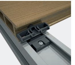
Výr. č. 9486 Montážna svorka pre systém Terrace vhodná pre všetky hliníkové nosné profily
