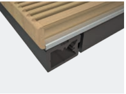
Výr. č. 9482 Ukončenie s koncovým krytom (len systém Terrace)
