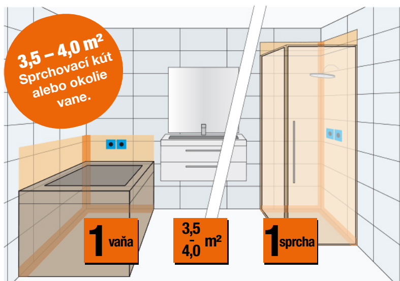
PCI Pecitape® 10x10 – izolácia prestupov PCI Pecitape® Objekt – izolácia kútov
