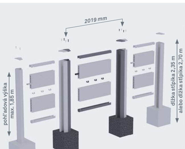
Súpravy P 9283 a P 9279: Zapustenie do betónu
