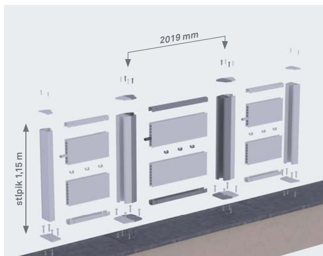
Súprava P 9282: Montáž na betónový základ
