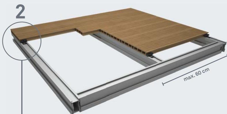
Hliníkový profil pre konštrukcie na nerovnom pevnom podklade 50 x 50 mm
